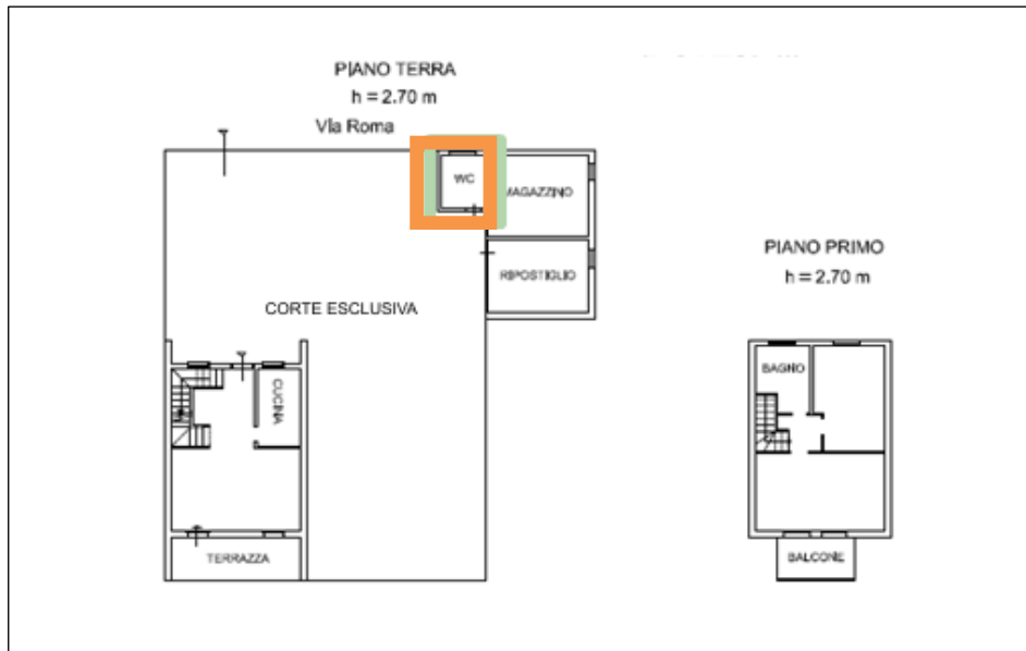
Figura 3.44: esempio di locale accessorio a servizio diretto di locali indiretti non comunicanti (poligono tipo C)
