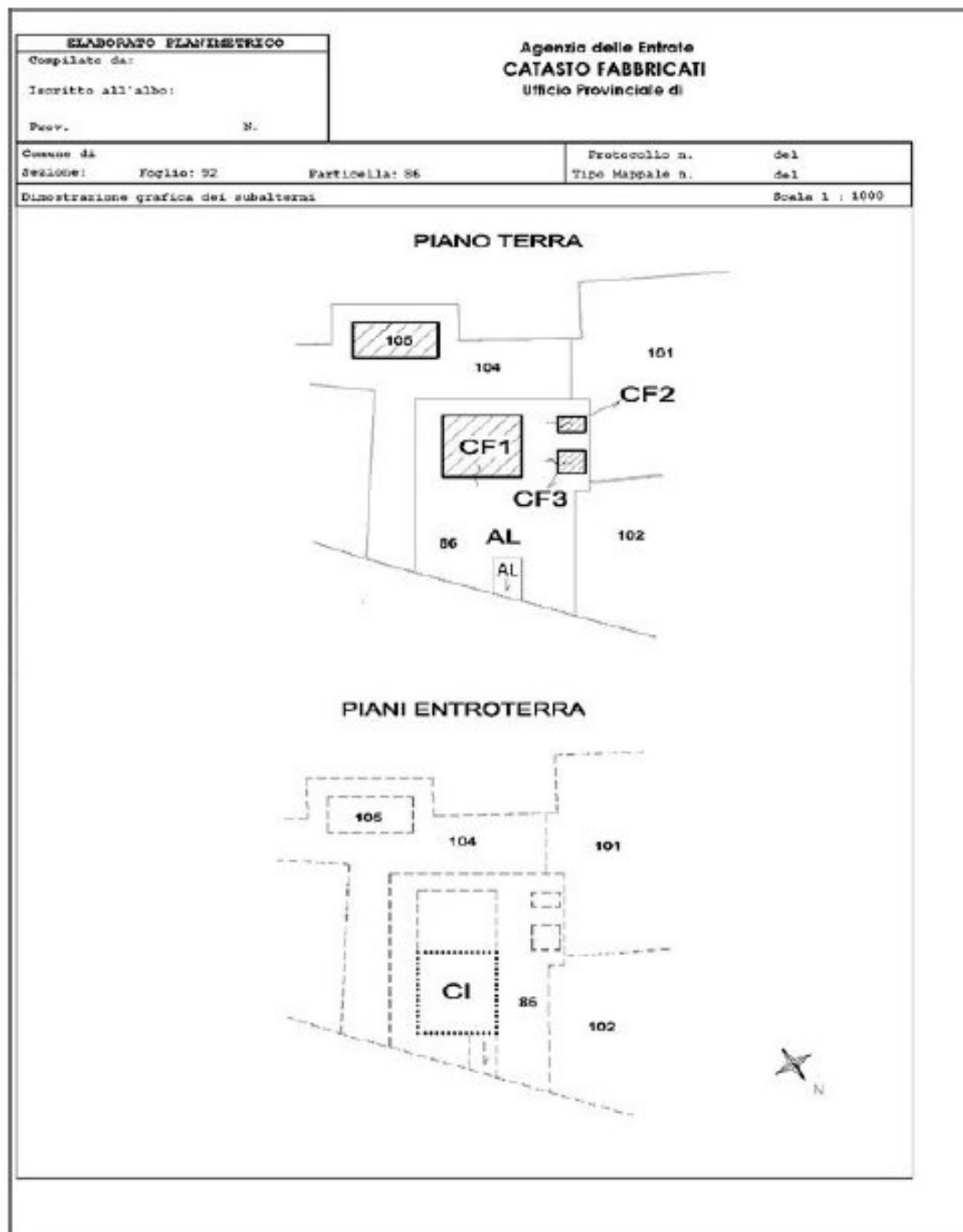
Figura 3.35: rappresentazione di elaborato planimetrico riportante le Entità tipologiche, CF (Costruzione di Fabbricato), AL (Area Libera), e CI (Costruzione Interrata), relative ad un edificio condominiale.
