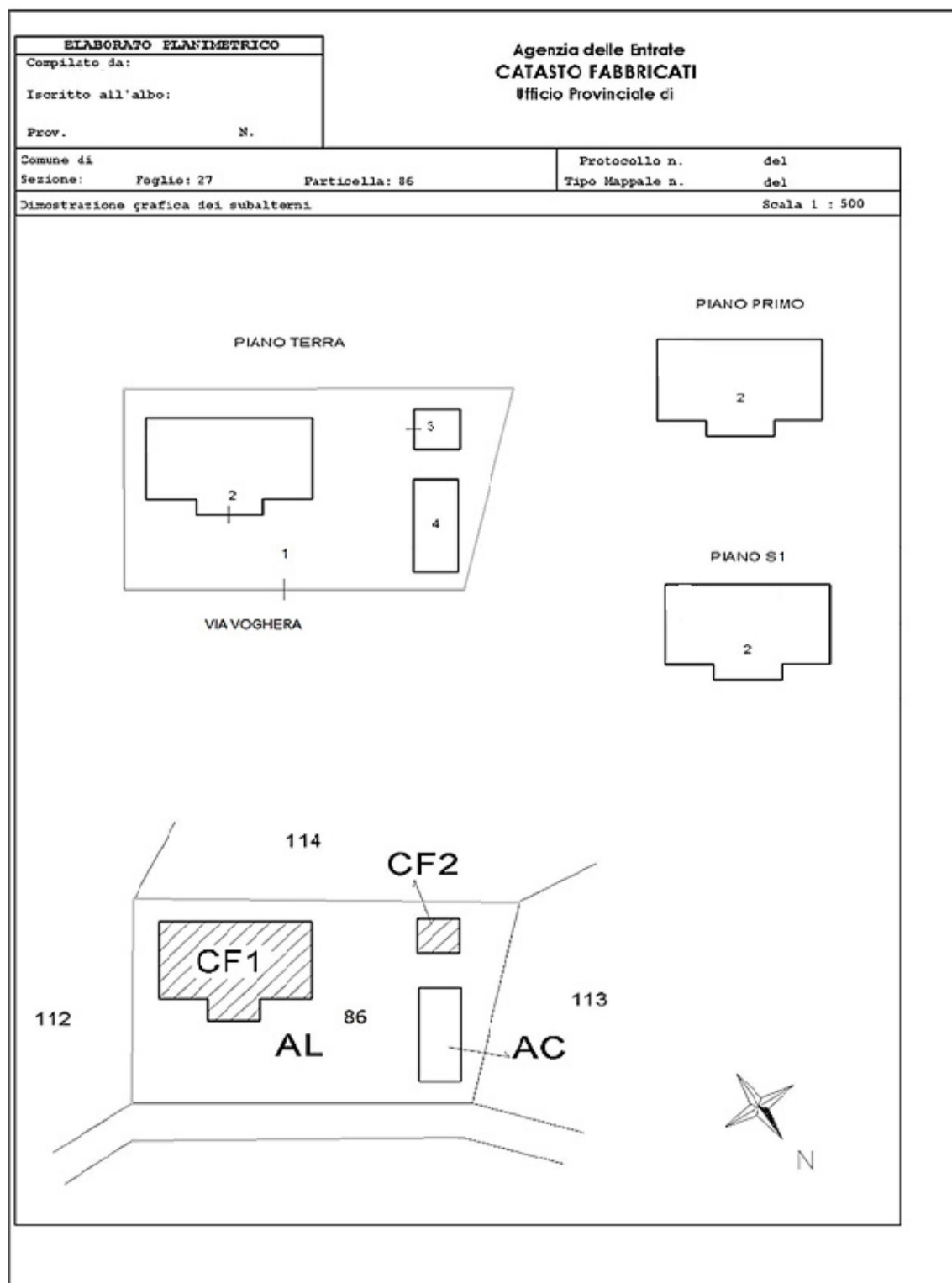
Figura 3.37: rappresentazione di un elaborato planimetrico riportante un fabbricato di nuova costruzione con una sola unità immobiliare a destinazione abitativa, una tettoia e un'autorimessa.
