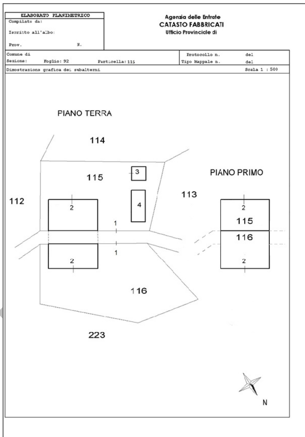
Figura 3.34: rappresentazione di elaborato planimetrico, di nuova costruzione, riportante il perimetro delle singole unità immobiliari e dei beni comuni non censibili, relativi alla Figura 3.33.
